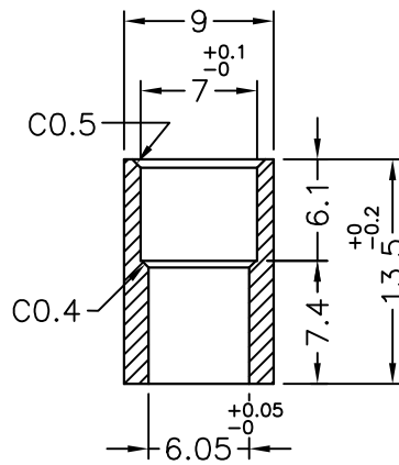
A-A 剖面
