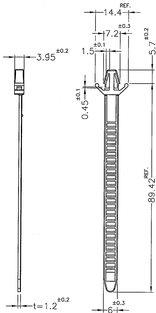
CABLE TIES SCALE 1:1
