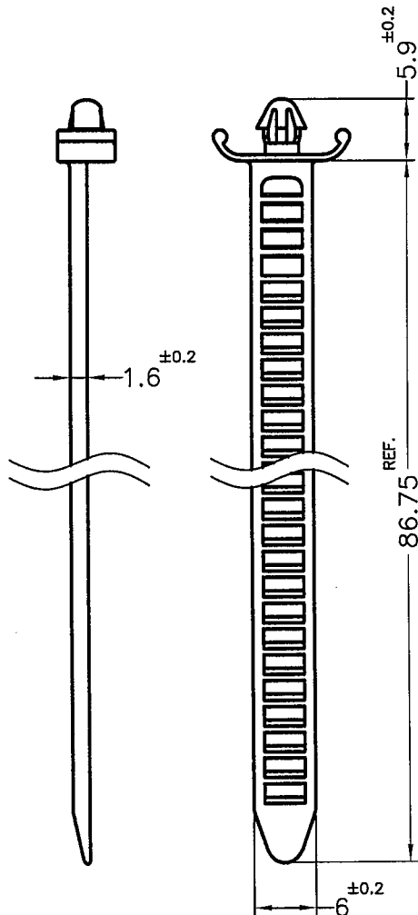
CABLE TIES SWPL-53B(B)
