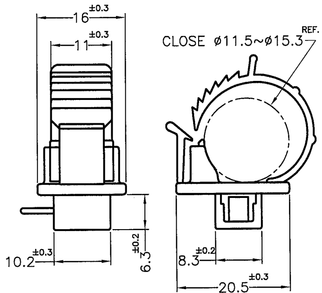
CABLE CLAMP SWPL-67A(B)
