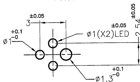
HOLE IN P.C.B
