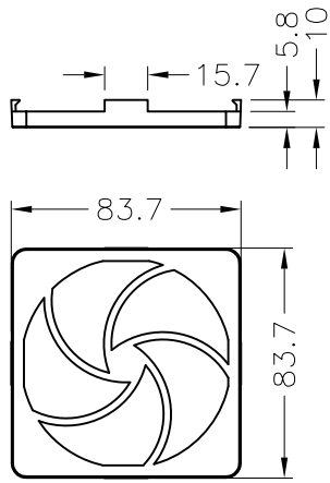
FANCV-5B
