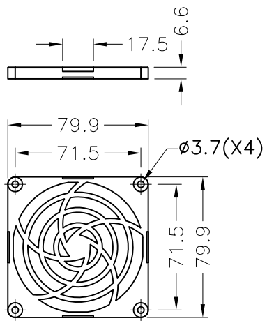
FANCV-5A
